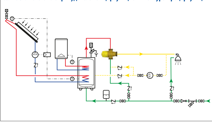
Солнечная система с принудительной циркуляцией и контуром рециркуляции
