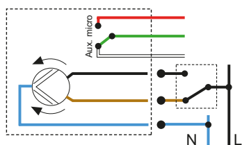
Электрическая схема M03.3 с 6 проводами со вспомогательным микропереключателем
